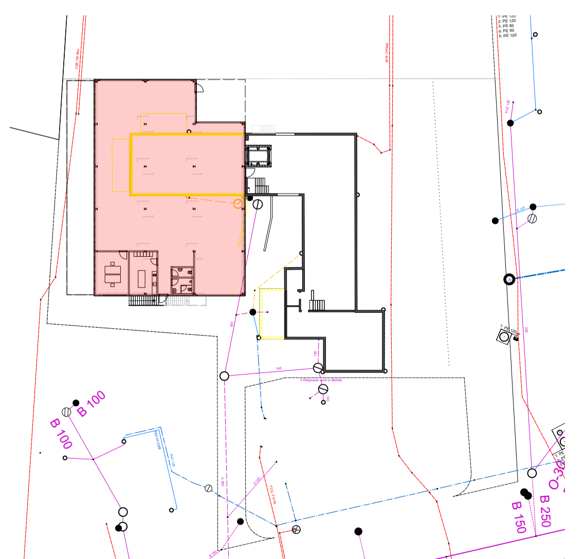
Grundriss UG
