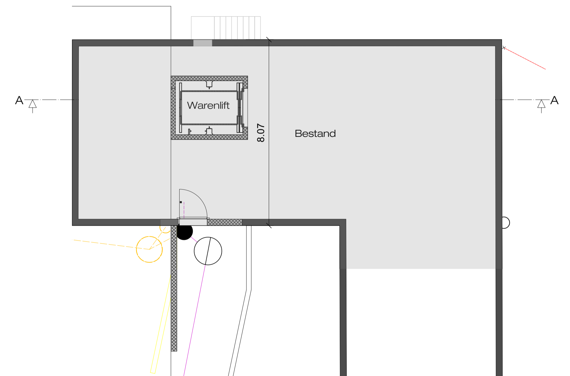
Grundriss UG
