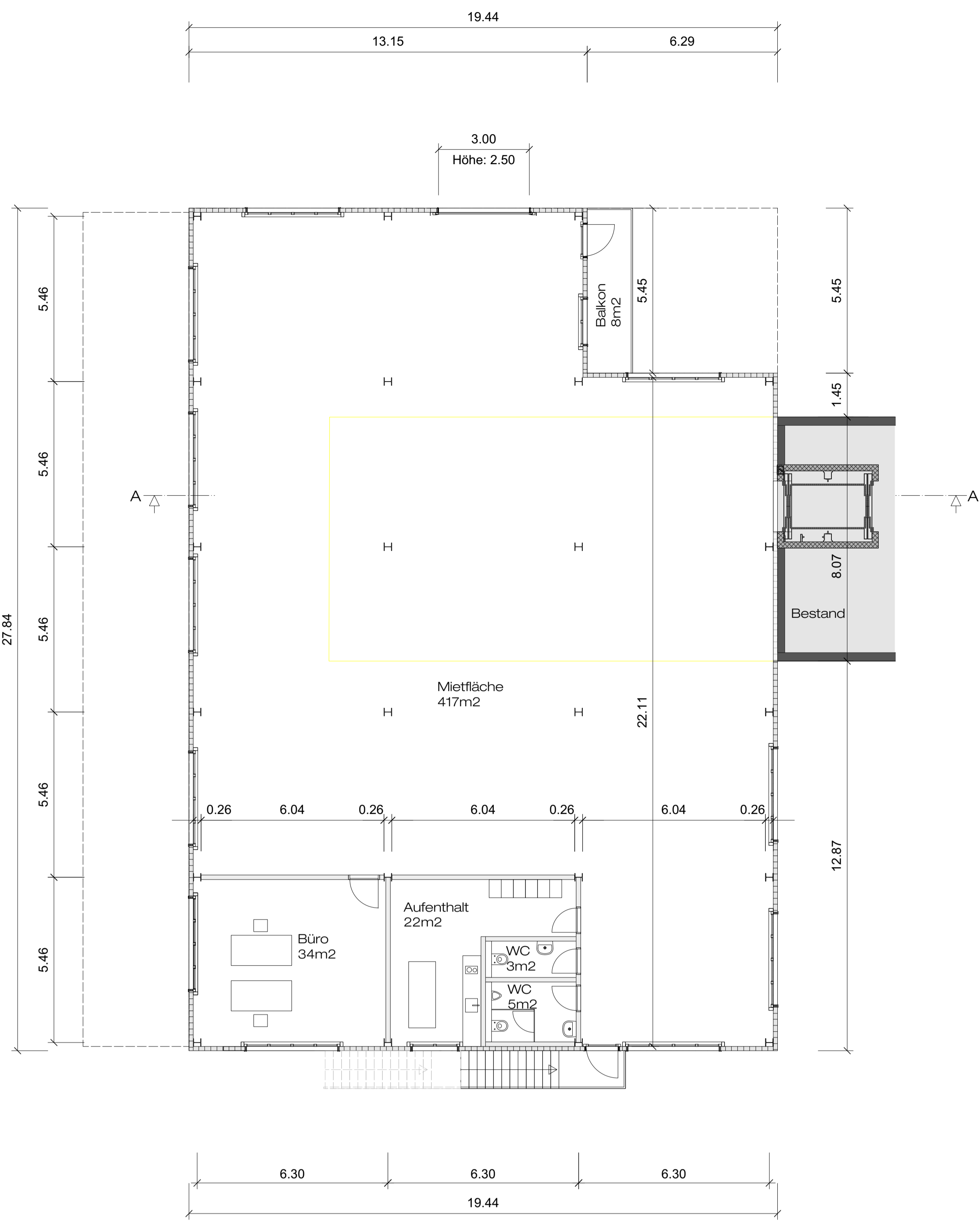
Grundriss 1.OG
