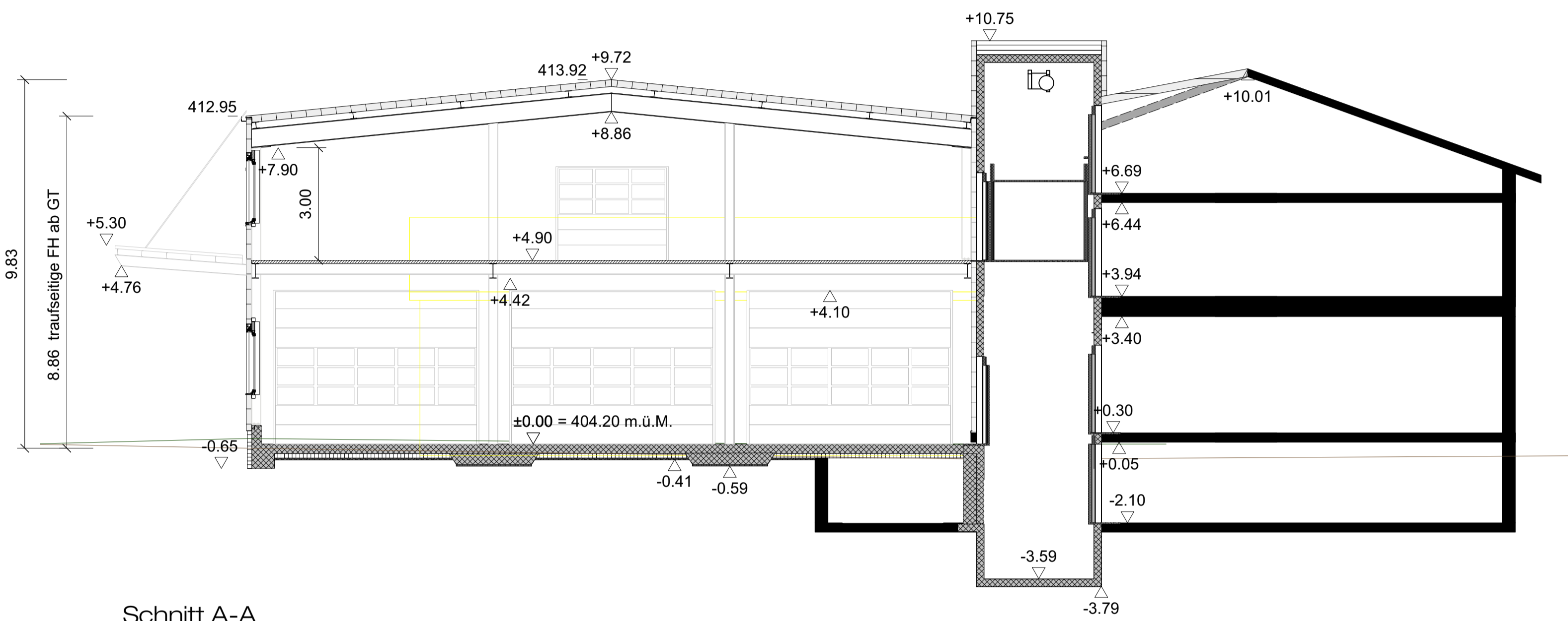
Schnitt A-A
